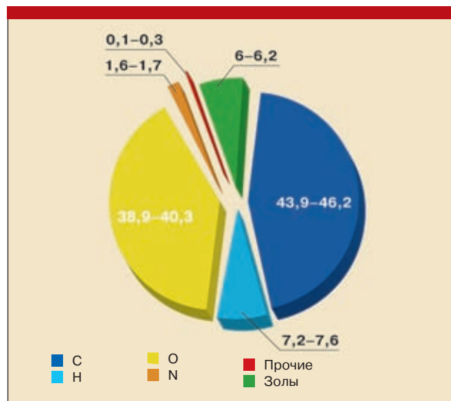
Рис. 4. Элементный состав органической субстанции российских ТБО, (% масс.)
